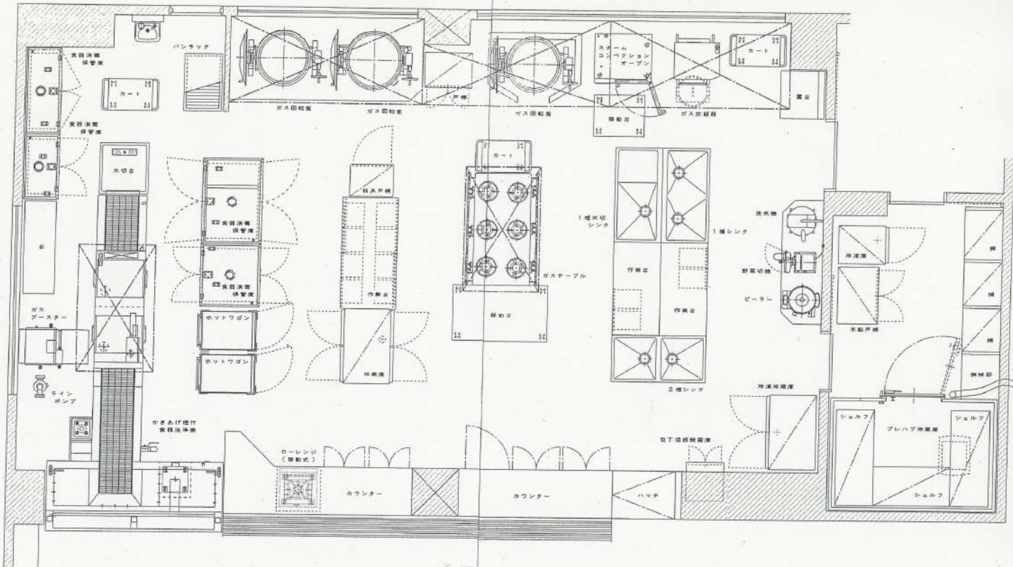
厨房機器平面図 松風園 殿 尺度: 1/30 H16.04.15
